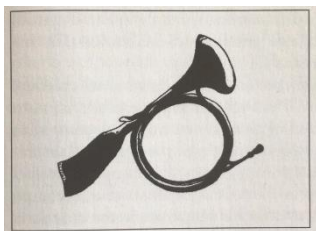
Figura 9 Figura chimerica
